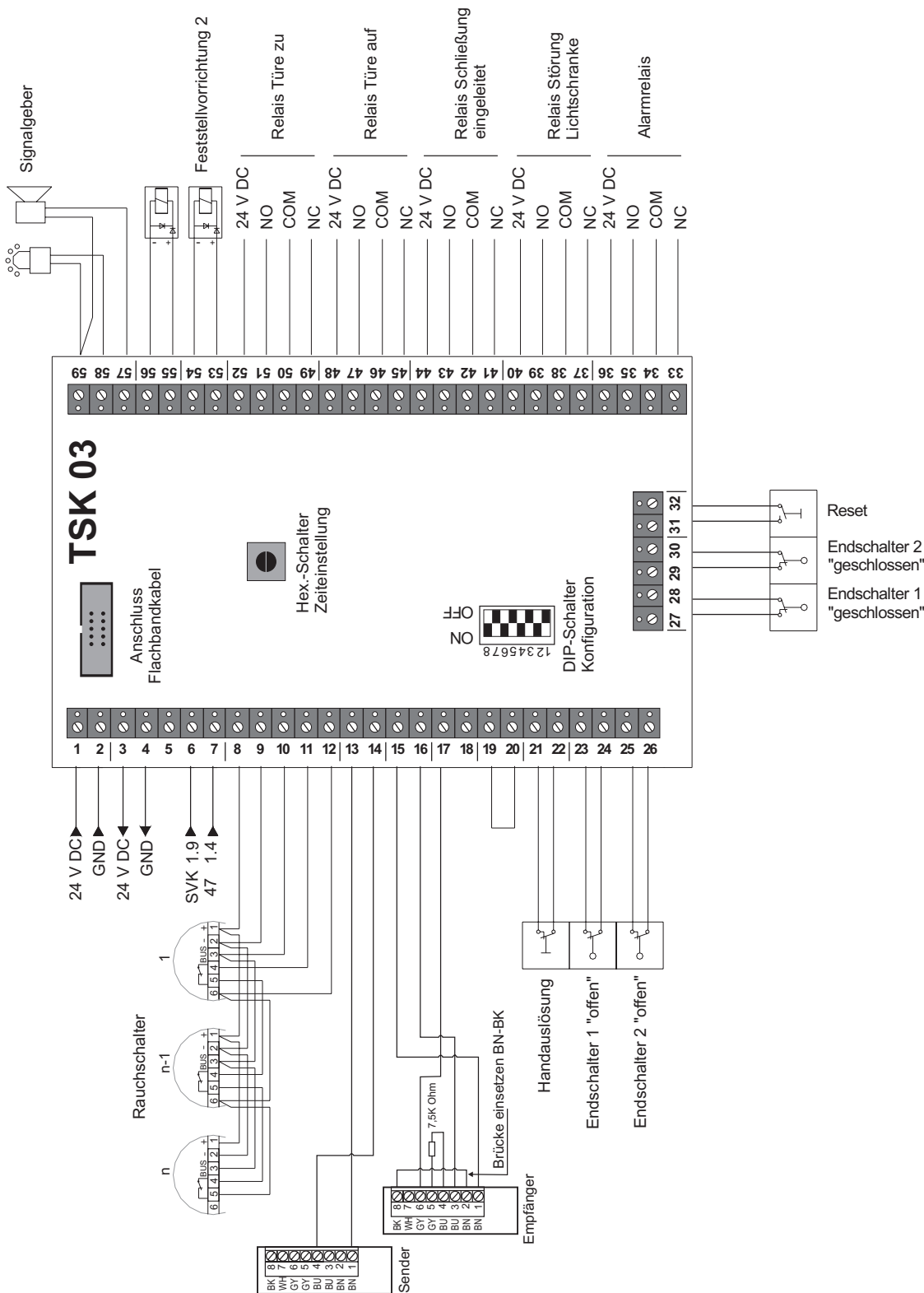
Abb. 6-5: Anschaltbeispiel der TSK 03 an einer Feststellanlage an bahngebundener Förderanlage
