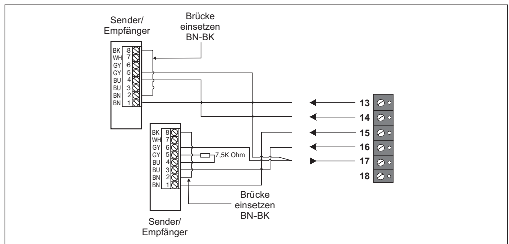
Abb. 6-15: Gruppenschaltung von 2 BRL-FSA/RLK 28-FC-55-2/31/116
