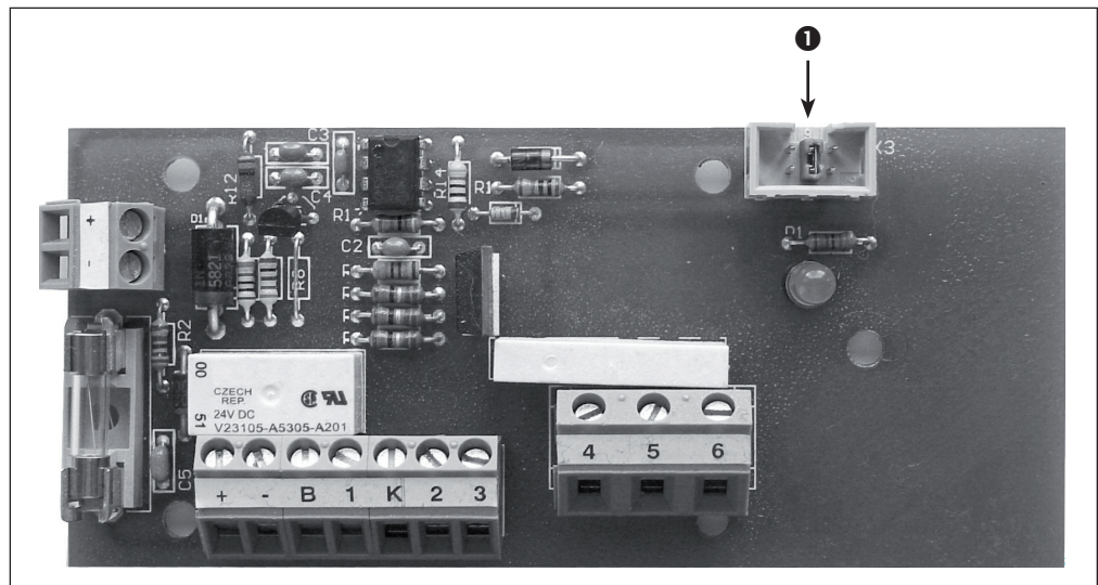
Abb. 3-6: Feststellanlagenkarte FAK 01/FAD 01
