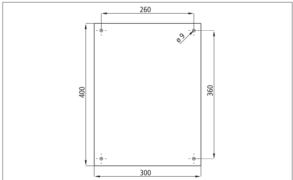
Abb. 5-3: Rückansicht SVG 522 ohne Befestigungslaschen
