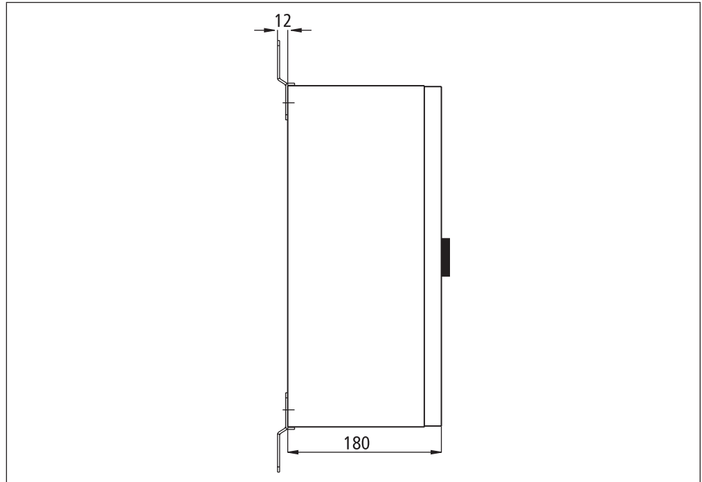
Abb. 5-2: Seitenansicht SVG 522 mit Befestigungslaschen
