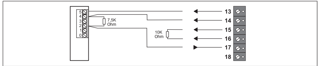
Abb. 6-12: RLS-FSA/RL24-55-2499 – Reflektionslichtschranke/Vorgänger-Lichtschranke zu BRL
