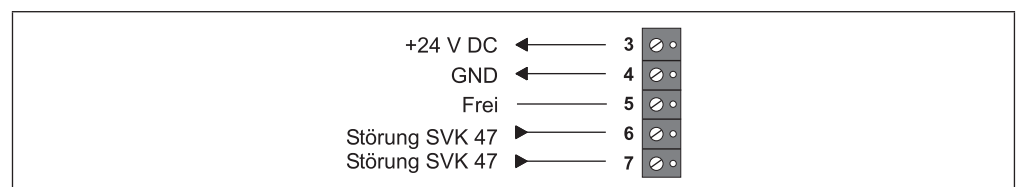
Abb. 6-7: Anschlüsse sind werkseitig verdrahtet
