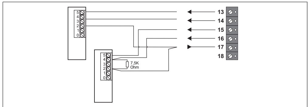
Abb. 6-14: Gruppenschaltung von 2 RLS-FSA/RL24-55-2499/Vorgänger-Lichtschranke zu BRL
