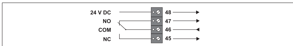
Abb. 6-34: Funktionsstellung in Zustand „Tür auf“ durch Endschalter
