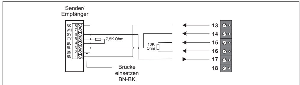
Abb. 6-13: BRL-FSA/RLK 28-FC-55-2/31/116 – Reflektionslichtschranke
