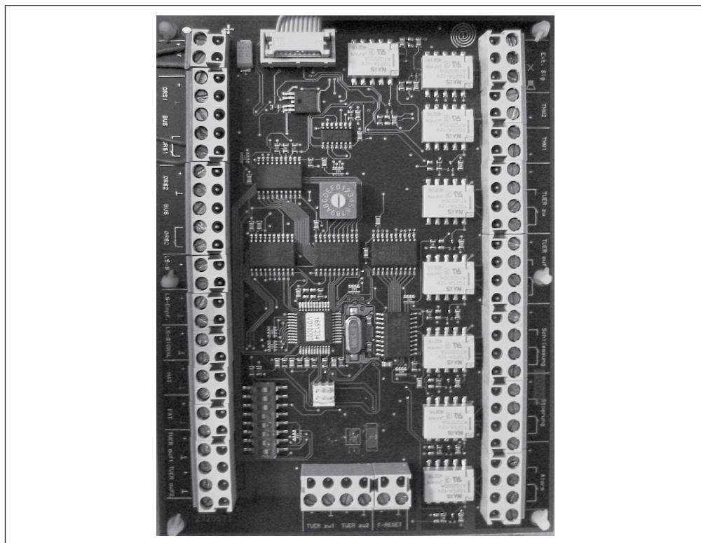
Abb. 3-5: Platine Türsteuerkarte TSK 03
